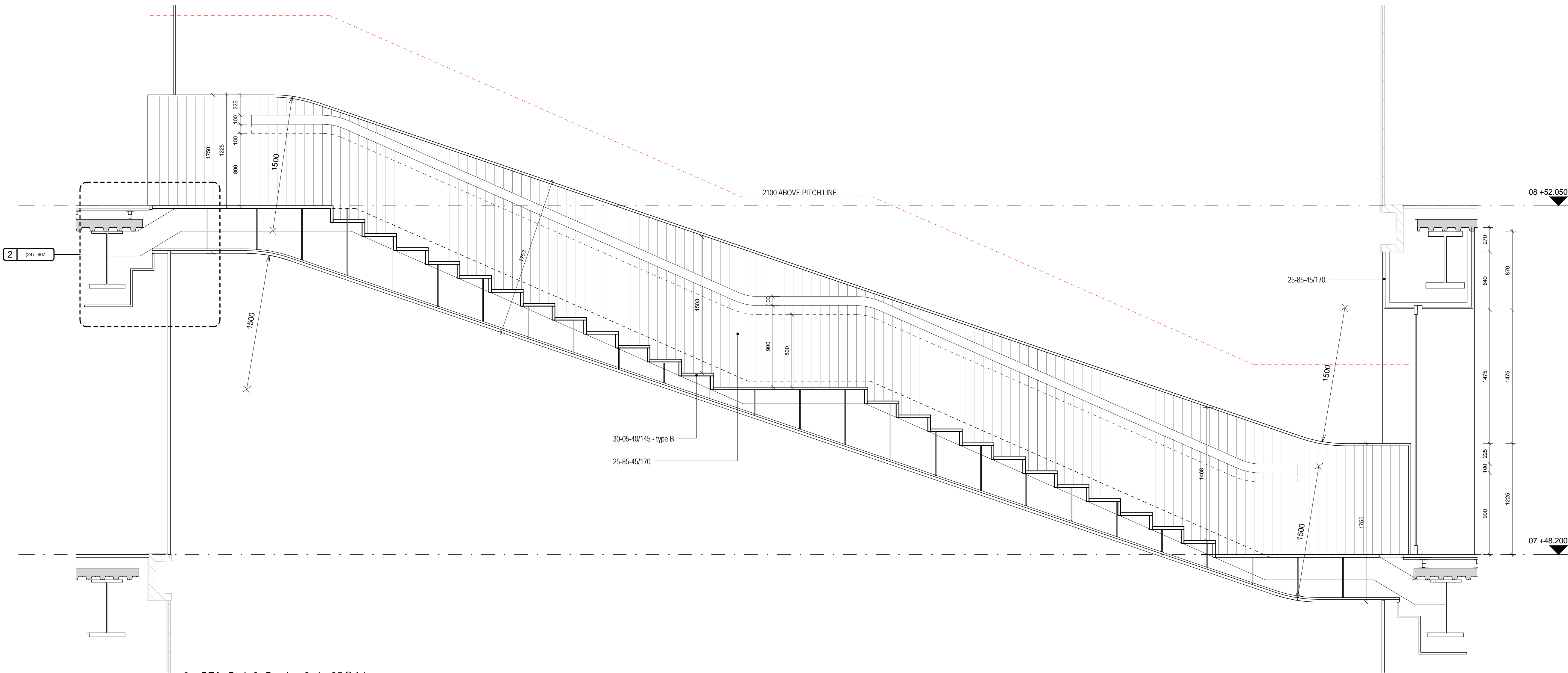
2 SFA_Stair 3 Section 2, 1 : 25@A1
